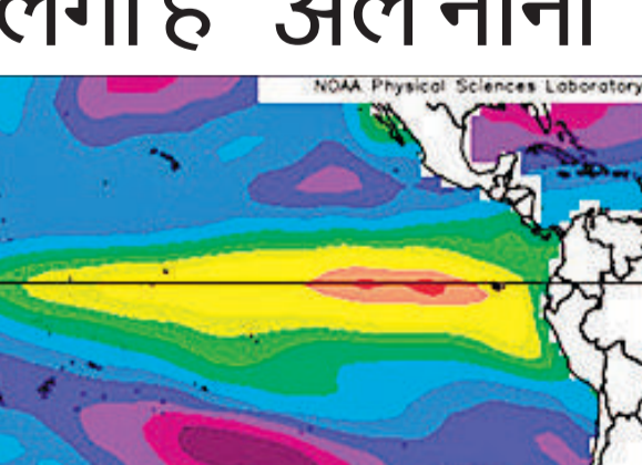
अल नीनो प्रभावित क्षेत्र का मानचित्र।
