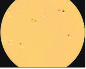
सूर्य की सतह पर उभरे सन स्पॉट।
