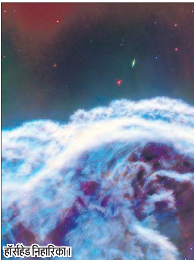
हॉर्सहेड निहारिका।
