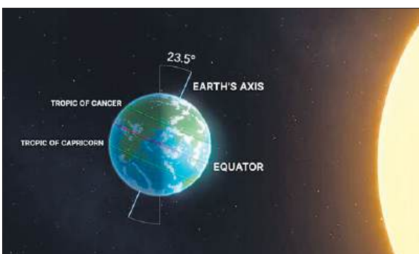
पृथ्वी पर दिन व रात का चित्र।
